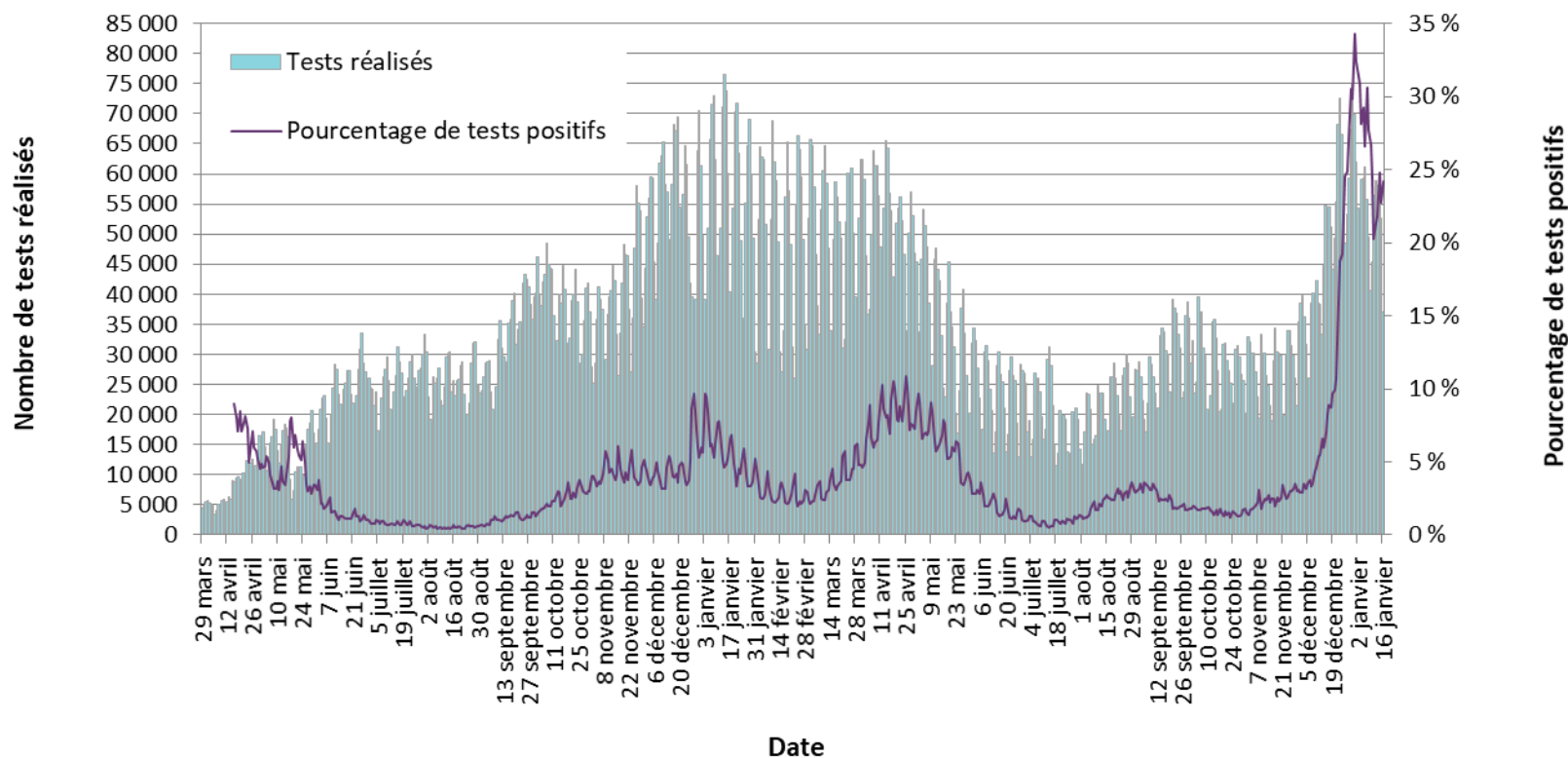
Figure 2 : Nombre de tests de dépistage de la COVID-19 effectués et pourcentage de tests positifs : Ontario, du 29 mars 2020 au 16 janvier 2022
