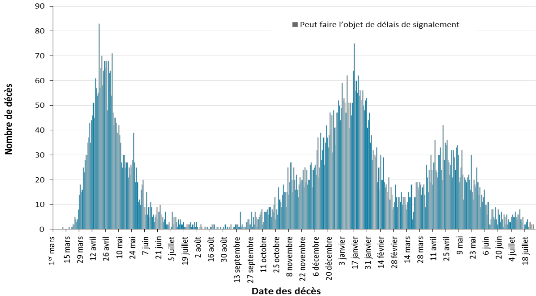
Figure 4 : Nombre de décès confirmés parmi les cas de COVID-19 selon la date des décès : Ontario, du 1 er mars 2020 au 29 juillet 2021
