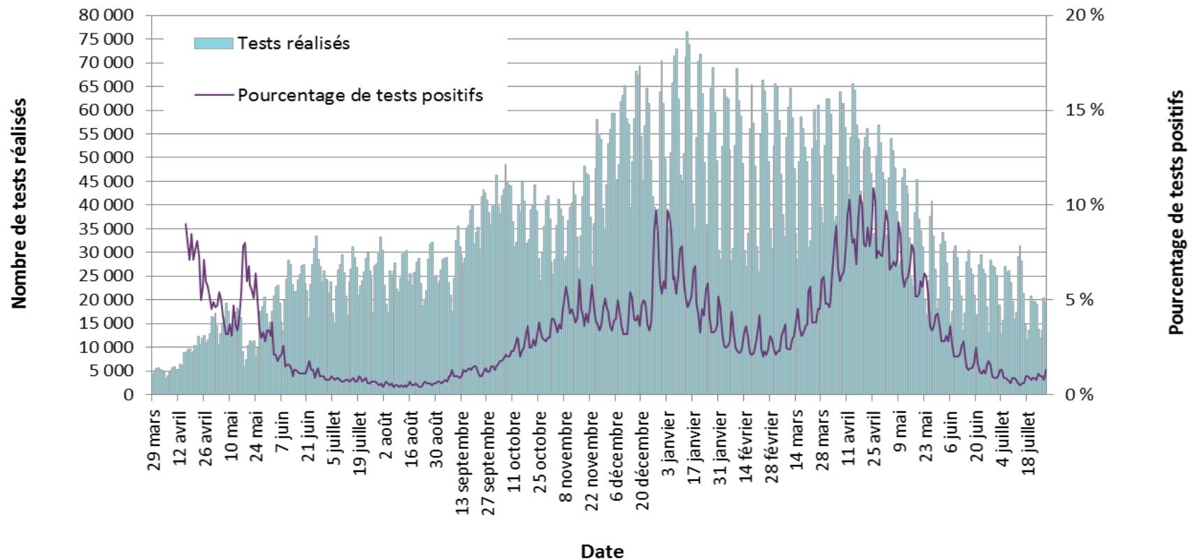
Figure 3 : Nombre de tests de dépistage de la COVID-19 effectués et pourcentage de tests positifs : Ontario, du 29 mars 2020 au 28 juillet 2021
