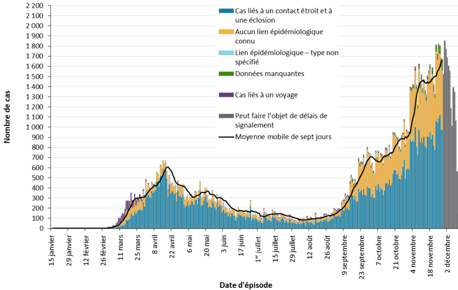
Figure 2 : Cas confirmés de COVID-19 selon la date probable d’infection et la date approximative d’apparition des symptômes : Ontario, du 15 janvier 2020 au 12 décembre 2020
