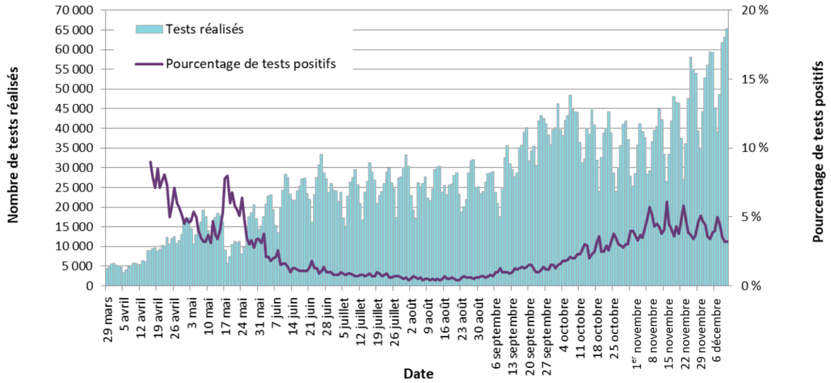
Figure 3 : Nombre de tests de dépistage de la COVID-19 effectués et pourcentage de tests positifs : Ontario, du 29 mars 2020 au 11 décembre 2020
