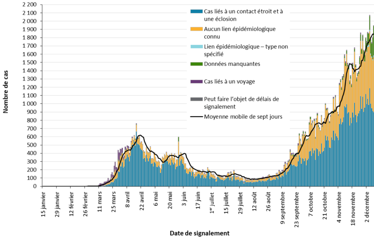
Figure 1 : Cas confirmés de COVID-19 selon la date probable d'infection et la date de signalement à un bureau de santé publique : Ontario, du 15 janvier 2020 au 12 décembre 2020
