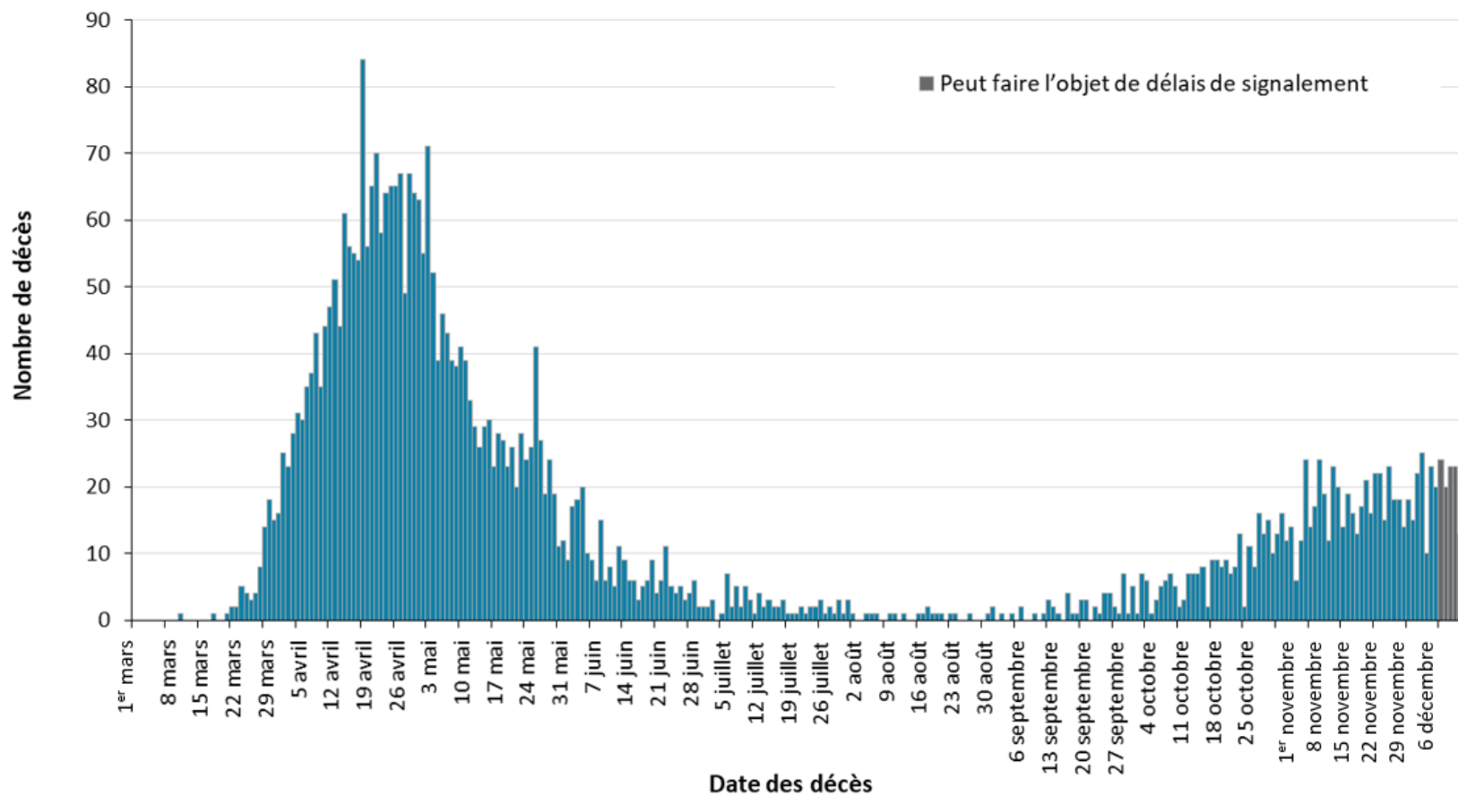
Figure 4 : Nombre de décès confirmés parmi les cas de COVID-19 selon la date des décès : Ontario, du 1 er mars 2020 au 12 décembre 2020
