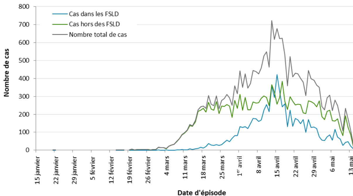
Figure 2 : Cas confirmés (n=22 311 1 ) de COVID-19 selon la date 2 approximative de l'apparition des symptômes par rapport à la situation dans les foyers de soins de longue durée (FSLD) 3 : Ontario, du 15 janvier 2020 au 15 mai 2020 4
